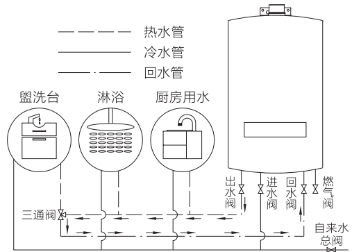
三管安装 图（2）
