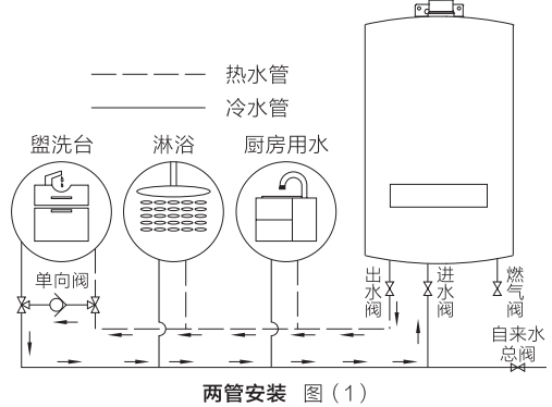
两管安装 图（1）
